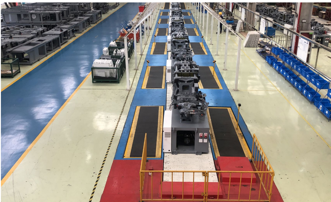
申达机器公司厂区数字化装配流水线
